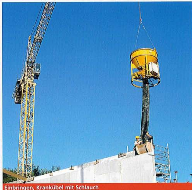
Einbringen, Krankübel mit Schlauch
